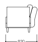
側面図 (ひじせを背として使用時)
