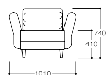
1P座+ひじせ+背クッション 正面図
