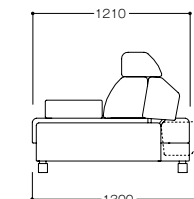
側面図
