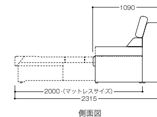
側面図
